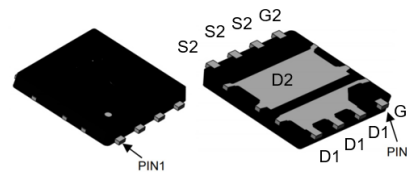
DFN5 x 6
